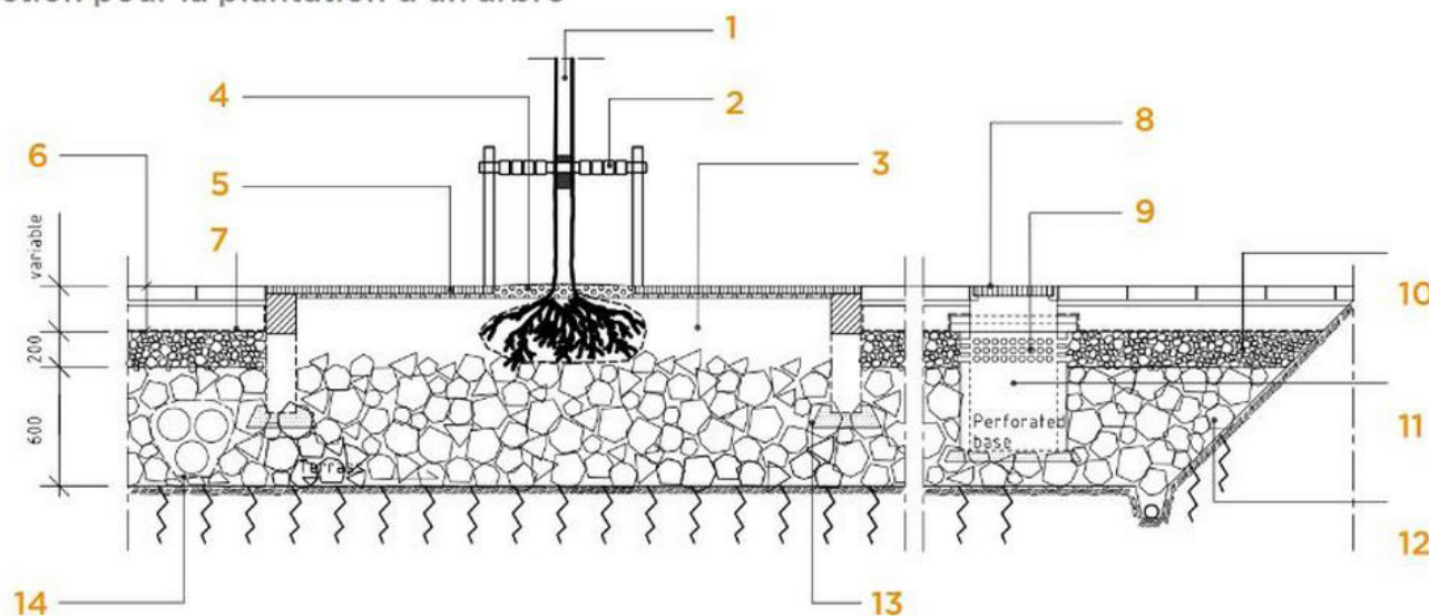
Schéma d'une tranchée de Stockholm
